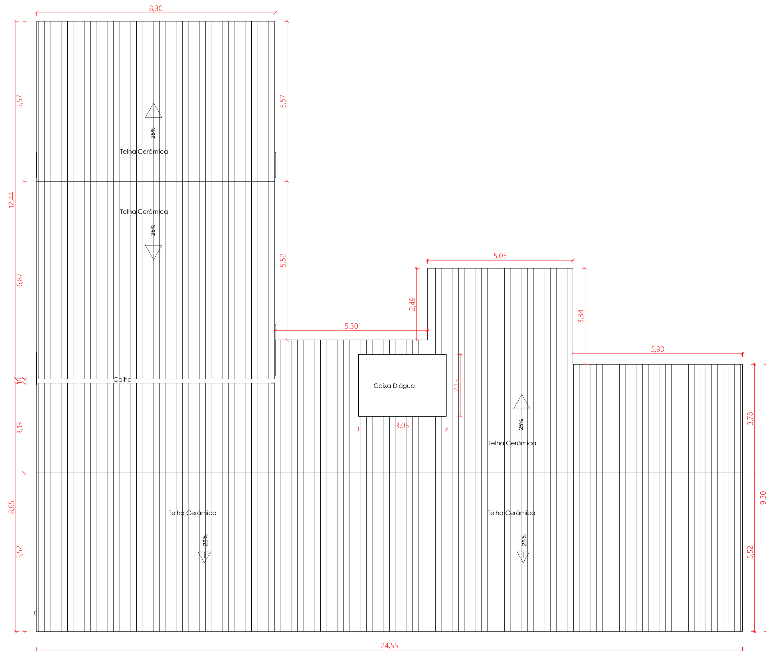
5 DIAGRAMA DE COBERTA ESCALA = 1 : 75
