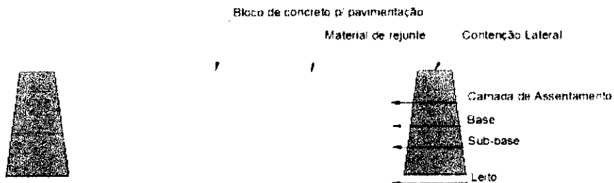
Imagem 15 – Processo executivo piso intertravado.
