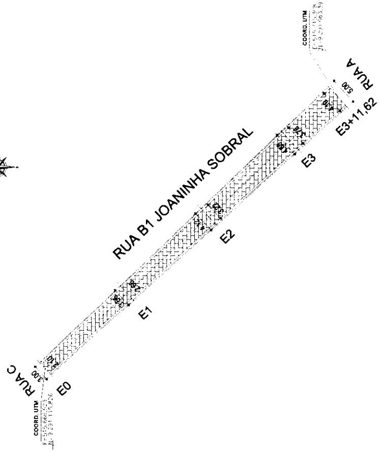
TOPOGRAFIA - ALINHAMENTO DA RUA ESCALA 1:200
