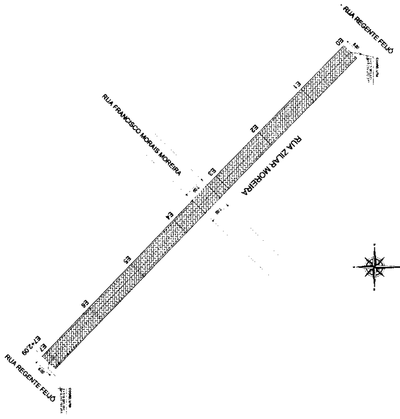
TOPOGRAFIA - ALINHAMENTO DA RUA ESCALA 1:400
