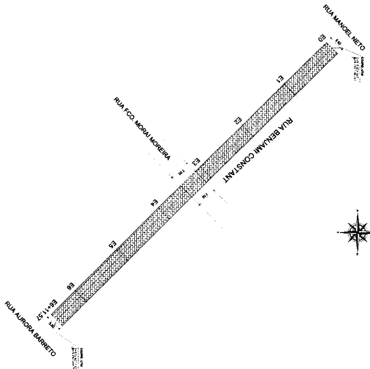
TOPOGRAFIA - ALINHAMENTO DA RUA ESCALA 1:400
