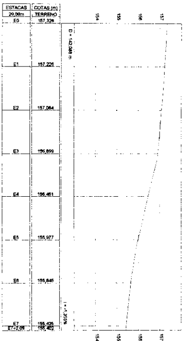
PERFIL DA RUA ESCALA 1:1000 V 10000
