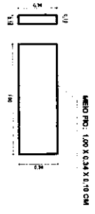
DETALHE DA GUA - MEIO FIO SEM ESC.
