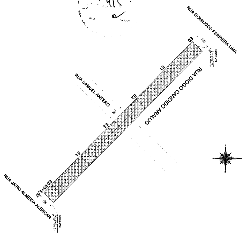
TOPOGRAFIA - ALINHAMENTO DA RUA ESCALA 1:400
