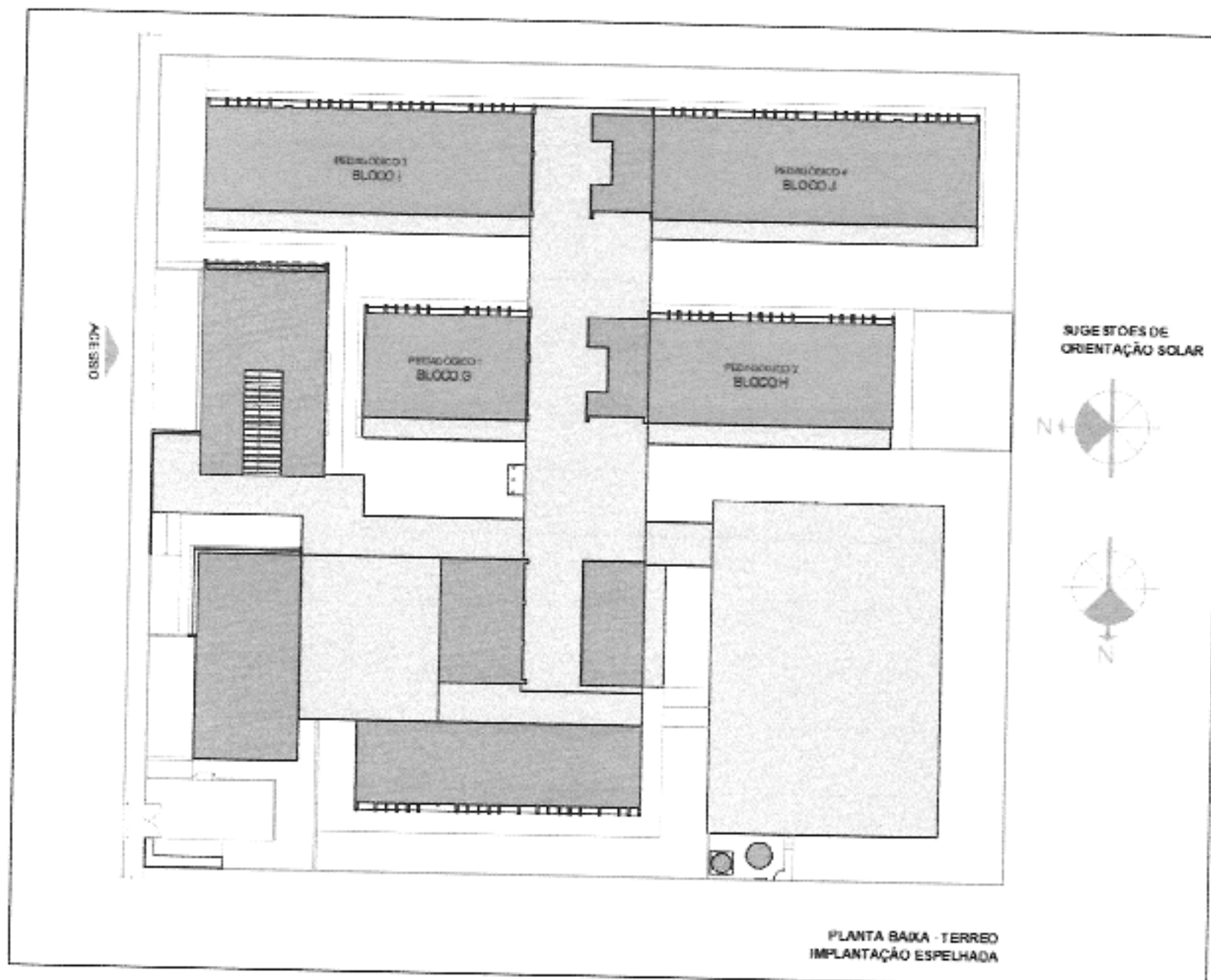
Figura 3 - croqui - implantação espelhada
