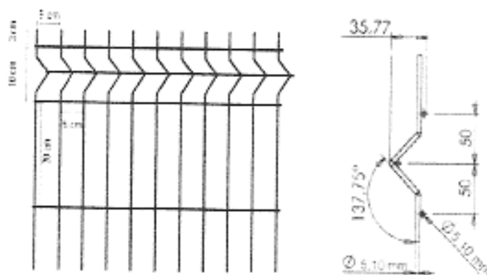
Figura 6 – imagem gradil morlan
