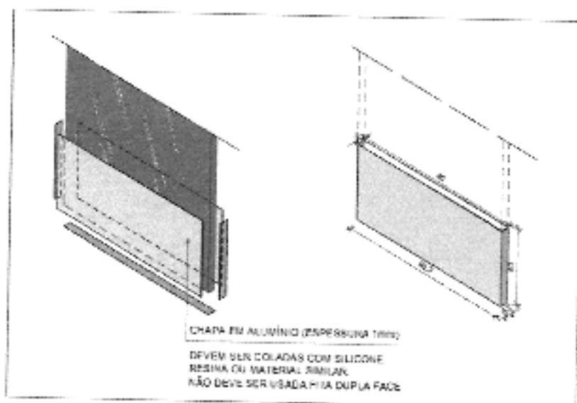
Figura 5 - detalhe chapa metálica para portas de madeira
