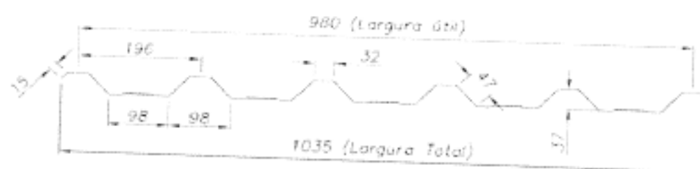
Figura 11 – imagem telha metálica trapezoidal TP40-980
