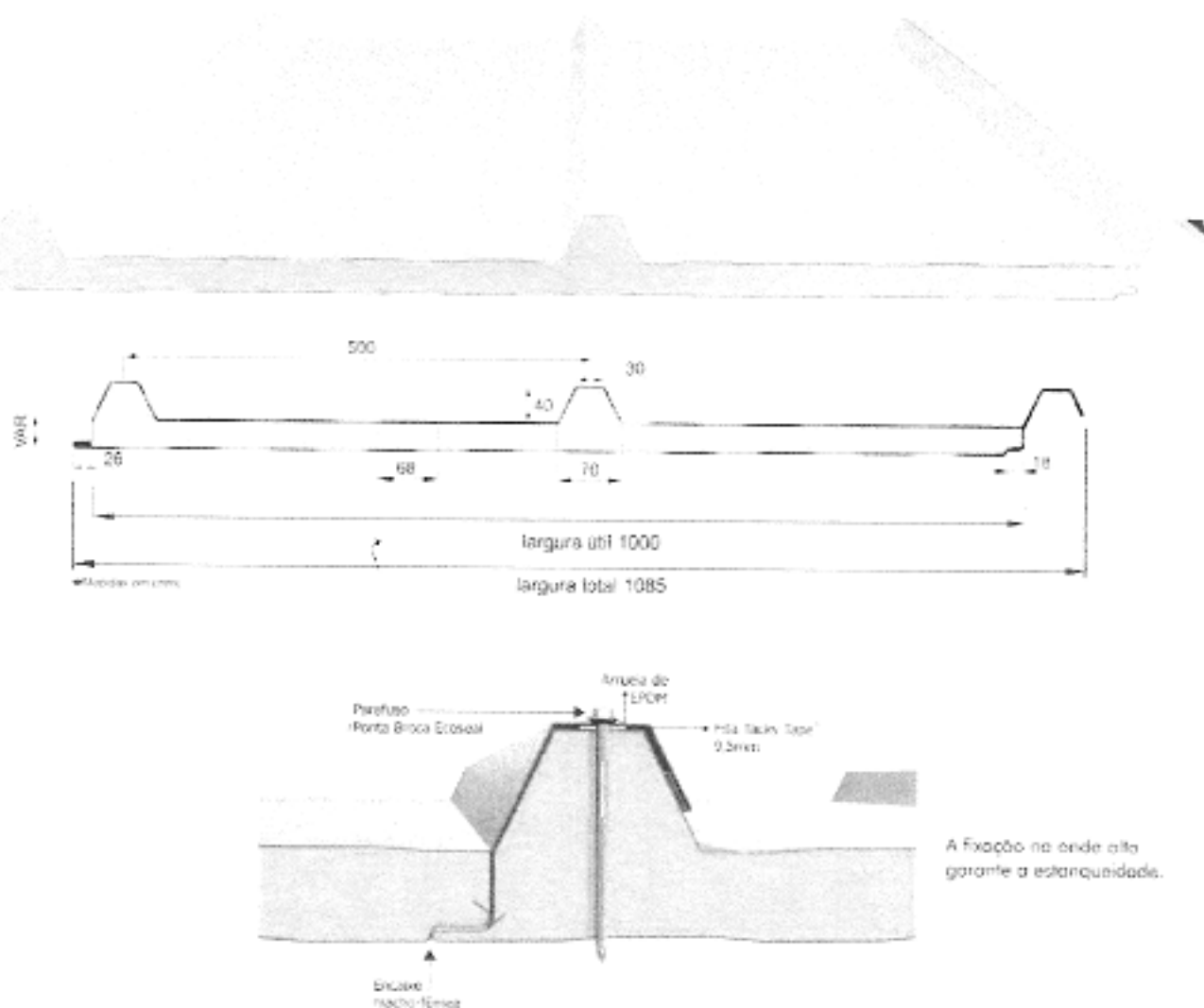
Figura 10 – imagem telha termoacústica
