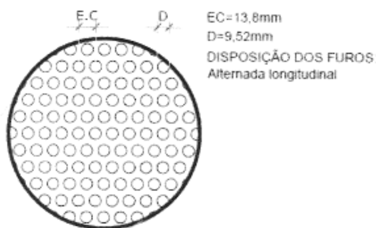
Figura 7 – imagem furos chapa metálica
