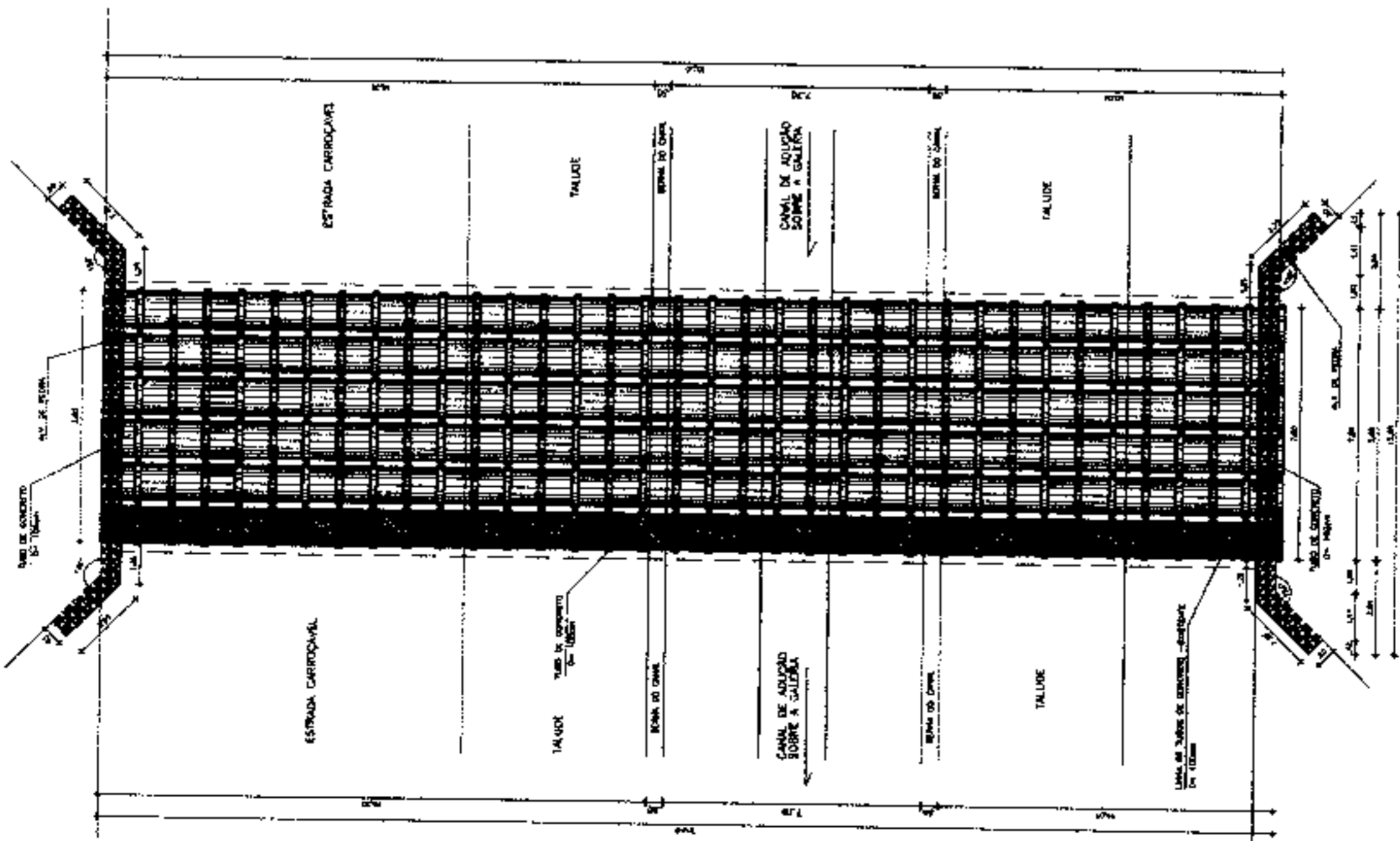
PIANTA BAIXA ESCALA 1:50
