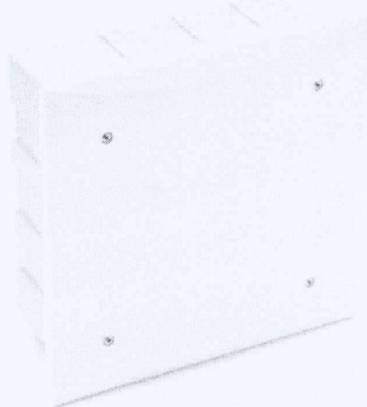
CAIXA DE PASSAGEM DE PAREDE, DE EMBUTIR, EM PVC, DIMENSOES *120 X 120 X 75* MM
