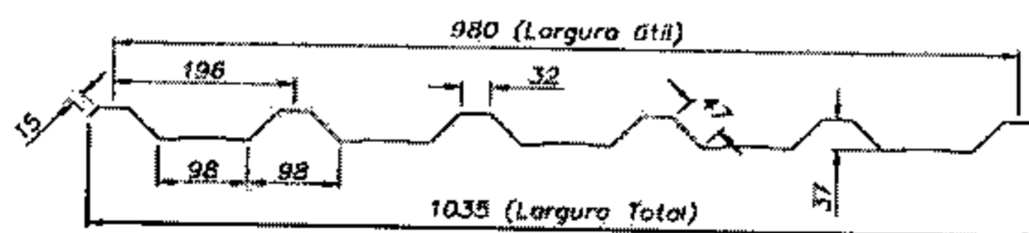
Figura 11 – imagem telha metálica trapezoidal TP40-980
