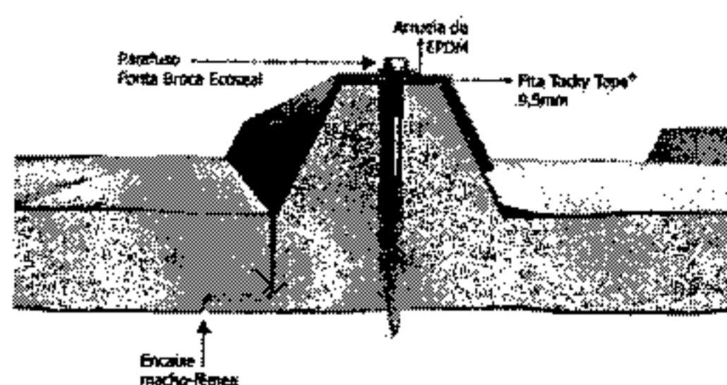
Figura 10 – imagem telha termoacústica
