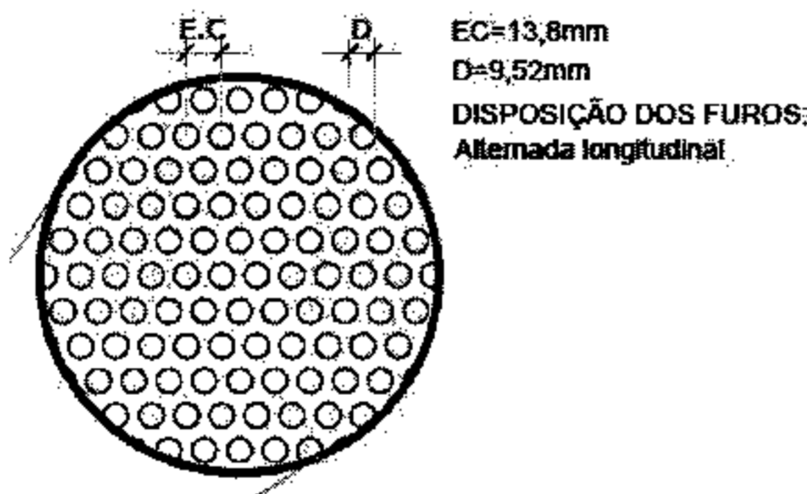
Figura 7 – imagem furos chapa metálica
